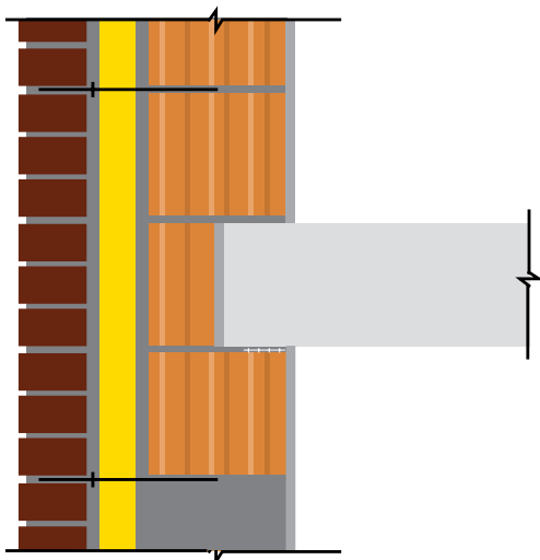
Несущая стена:
