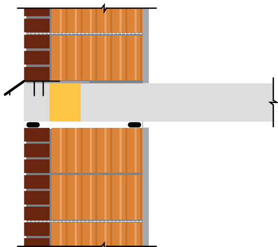
Монолитно-каркасная стена:
