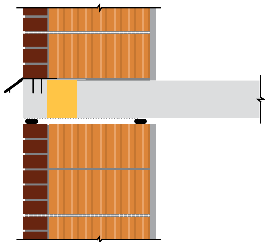
Монолитно-каркасная стена:
